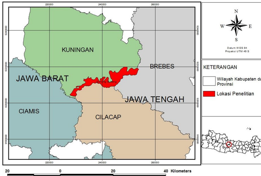
Gambar 1. Lokasi penelitian populasi surili di kelompok hutan Gunung Subang, Kabupaten Kuningan.
