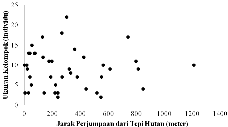
Gambar 2. Distribusi ukuran kelompok pada masing-masing jarak lokasi perjumpaan dari tepi hutan.
